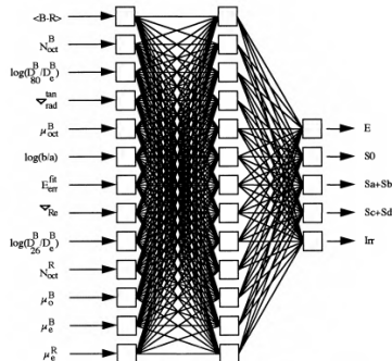
13 Galaxy Parameters Input Layer Hidden Layer Output Layer -> Classification
