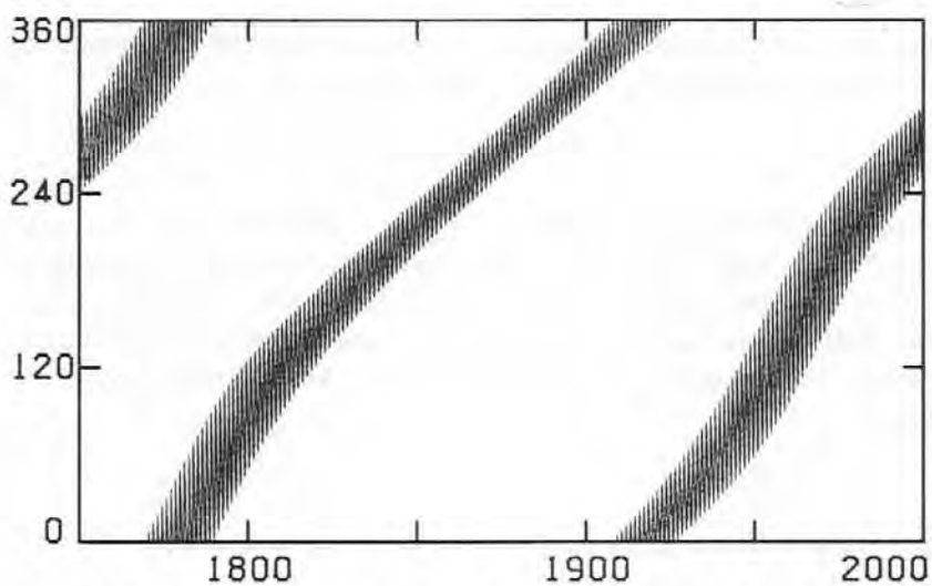
FIGURE 6.2 - PERIJOVE OF J3(GANYMEDE)
