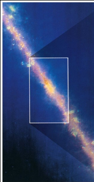
Infravermelho, campo de 50°.
