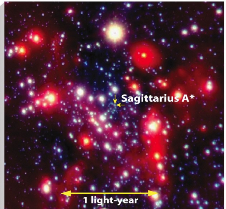
Zoom centrado em Sg A*, uma fonte de rádio bem no centro da VL, onde se observa centenas de estrelas próximas de Sagitário A* dentro de 1 al ou 0,3 pc.
