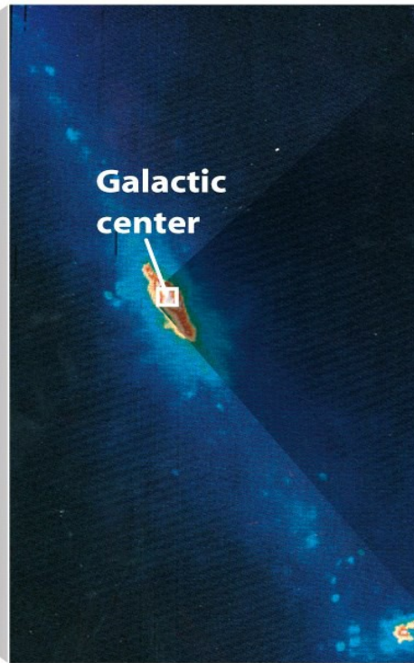
Infravermelho, com destaque ao centro Galáctico.
